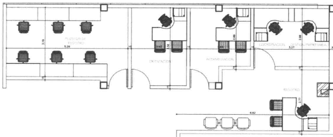
Figura 3. Planos Piso 2
